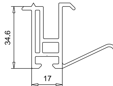
Подставочный профиль арт.№ 110054
