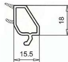
Штапик - арт. № 107140 (для стеклопакета 24 мм)
