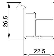
Подставочный профиль арт.№ 110001
