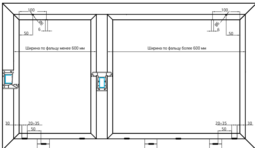
Отверстия в раме с импостом
