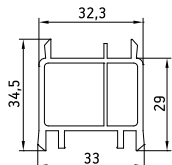
Соединитель-усилитель 014
