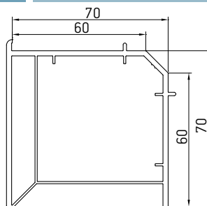
023 90° угловой соединитель 60/70
