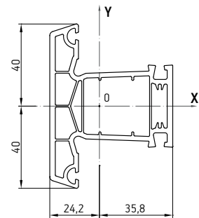
027 Импост
