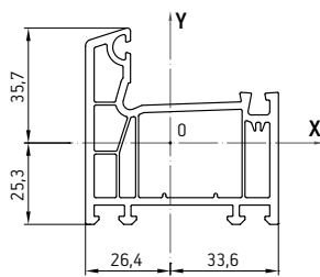
037 Рама
