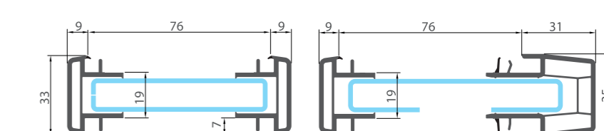
076 З'єднувач-підсилювач // I-connector
