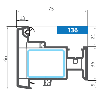
Штульп // Stulp
