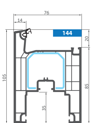
Стулка // Sash
