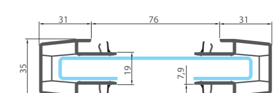
123 З'єднувач-підсилювач // I-connector
