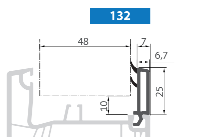
Штапики // Glazing beads
