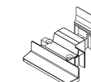
For 135 Металевий з'єднувач імпоста 76 AD // Metallic mullion connector 76 AD
