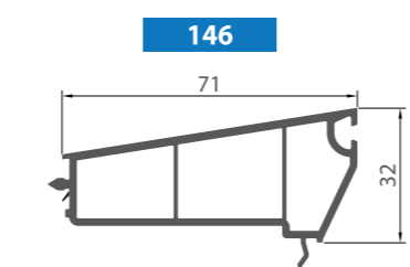
Заглушка стулки / / Cover profile for sash
