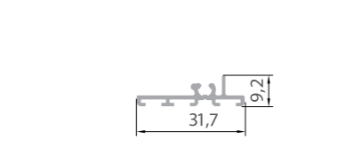
D000173 Профіль ущільнювача порога / / Threshold gasket profile
