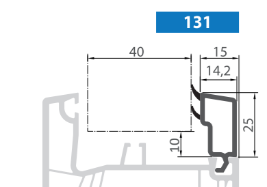
Штапики // Glazing beads
