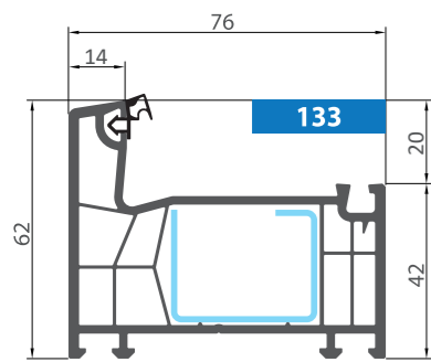
Рама // Frame
