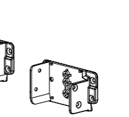
For 145 Металевий з'єднувач широкого імпоста 76 AD // Metallic wide mullion connector 76 AD
