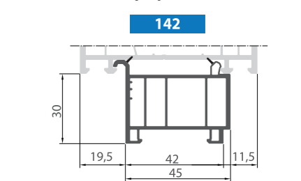
Листва // Platband
