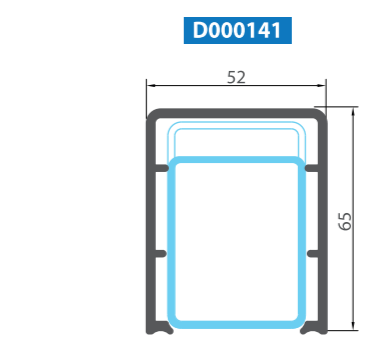
Накладка підсилення імпоста / / Reinforcement cover profile
