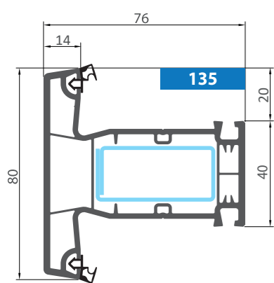
Імпост // Mullion
