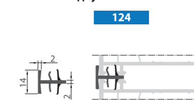
Н-з'єднувач // H-connector
