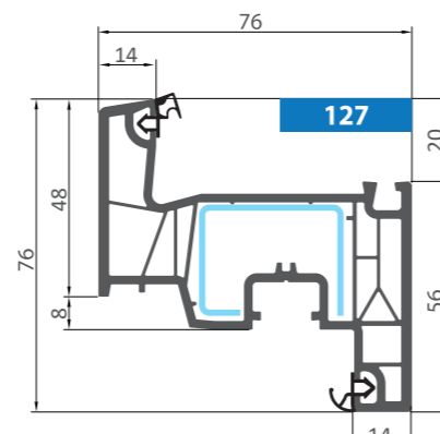
Штульп // Stulp
