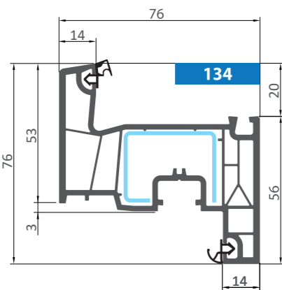
Стулка // Sash
