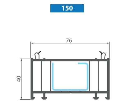
Розширювач рами // Frame extension
