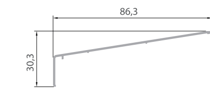
D000171 Алюмінієва кришка рами / / Aluminum frame cover
