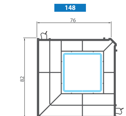
Кутовий з'єднувач // Corner adapter
